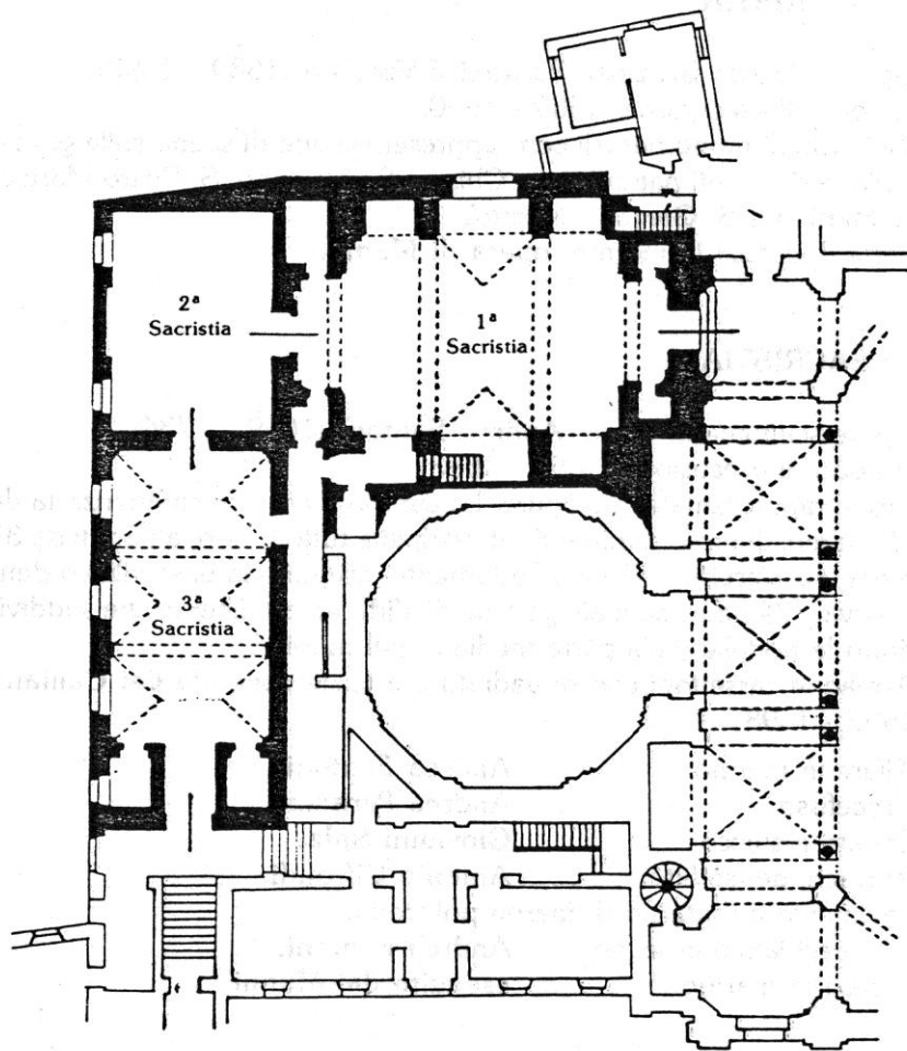
PIANTA SACRISTIE DELLA BASILICA S. MARTINO
